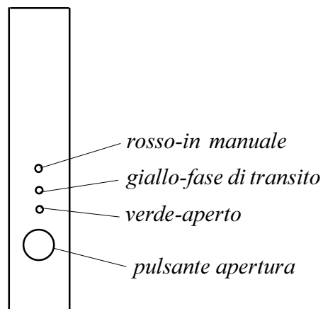
FIGURA 5 PULSANTIERA INT.
