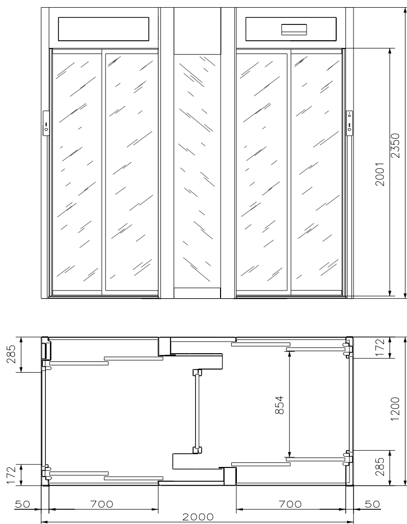
Lato esterno
