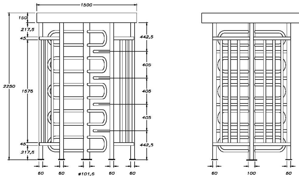
Габаритные размеры TR-104 SINGLE 3 sectors
