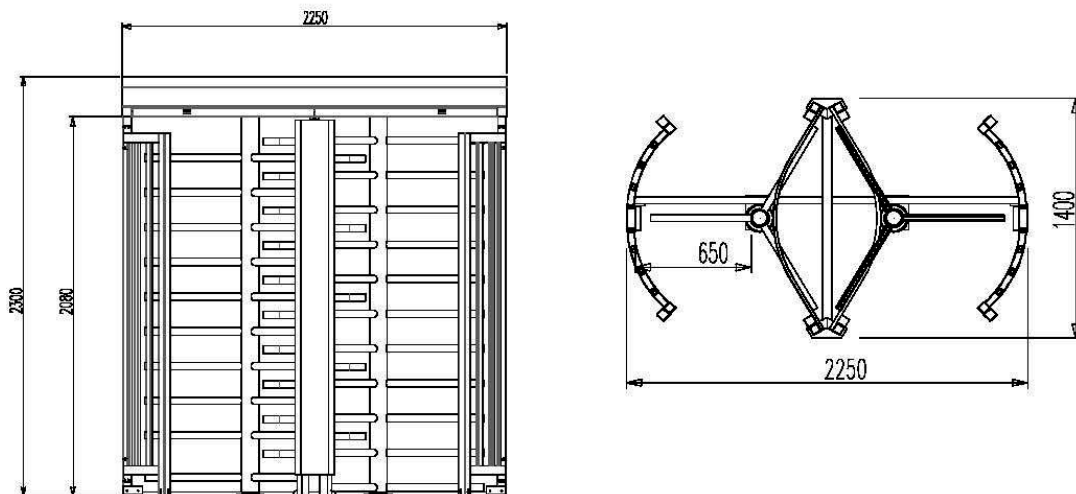
Габаритные размеры TR-121 DOUBLE 43 sectors
