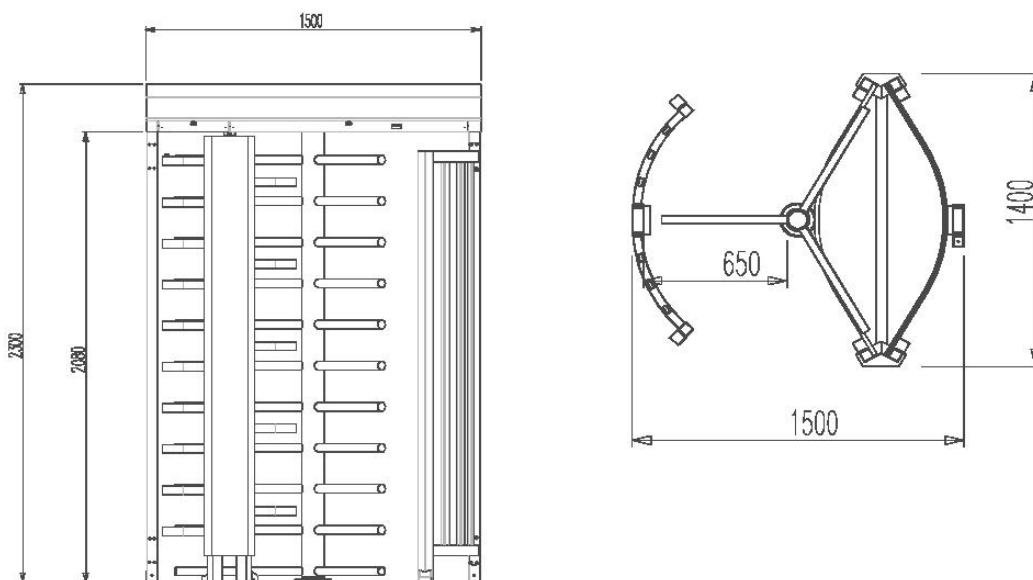
Габаритные размеры TR-121 SINGLE 3 sectors
